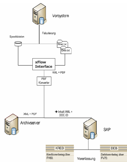
Abb.01 Ablaufschema
